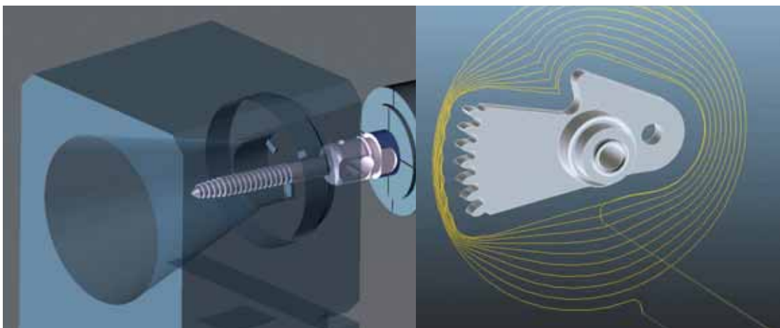
Simulation d'une opération de tourbillonnage pour la réalisation d'une vis à os.
